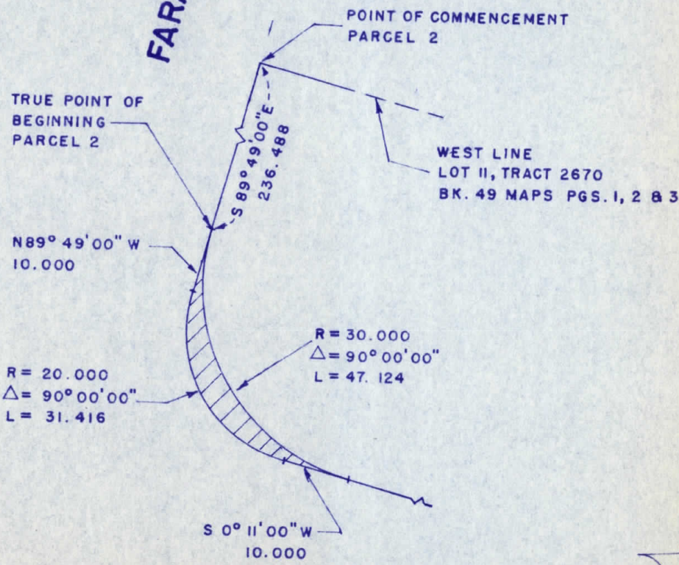
PARCEL 2 DETAIL
